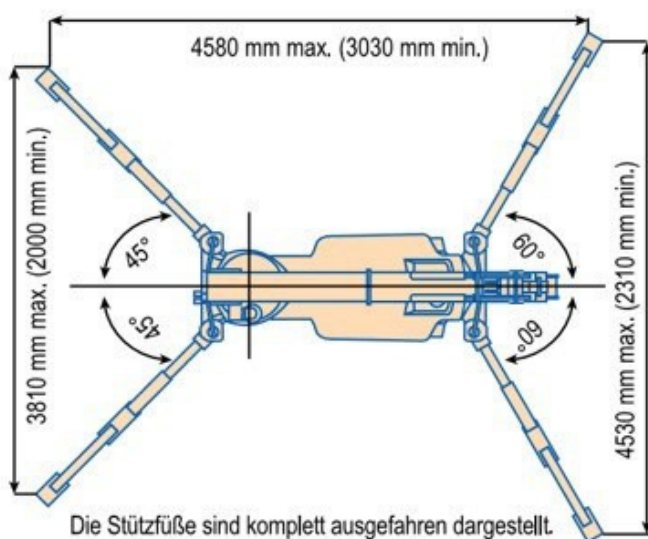
Abmessungen bei ausgefahrenen Stützfüßen
